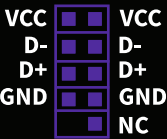
Conector USB 2.0 da Placa-Mãe
