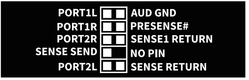
Conector de Áudio HD da Placa-Mãe
