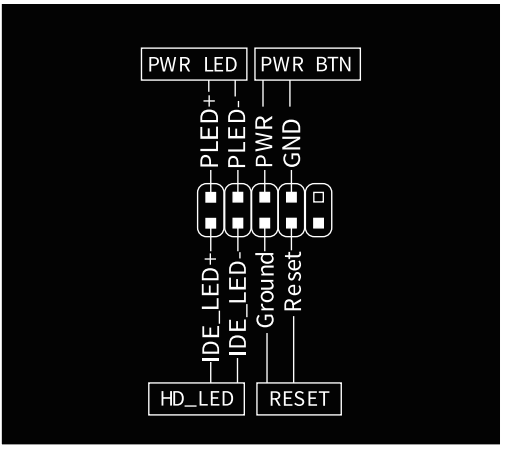
Conector Power/Reset/LED da Placa-Mãe
