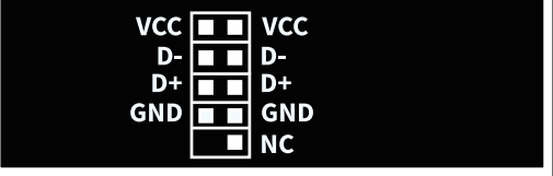
Conector USB 2.0 da Placa-Mãe
