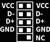
Conector USB 2.0 da Placa-Mãe
