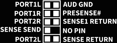
Conector de Áudio da Placa-Mãe
