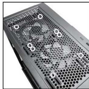
Fixe os parafusos na parte de fora da parte superior do gabinete
