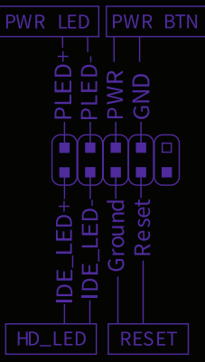
Conector Power/Reset/LED de la Placa Madre
