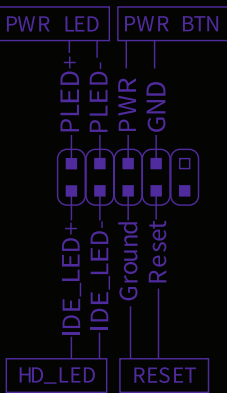
Conector Power/Reset/LED da Placa-Mãe
