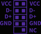
Conector USB 2.0 da Placa-Mãe
