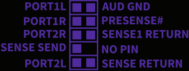
Conector de Áudio HD da Placa-Mãe
