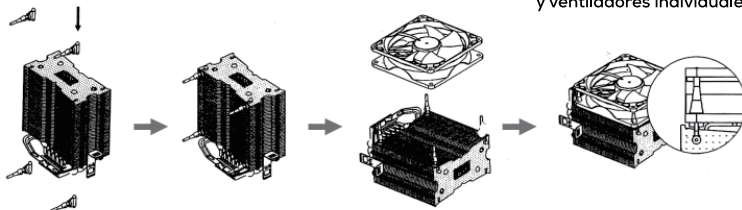
Tornillos para el soporte de montaje Intel
