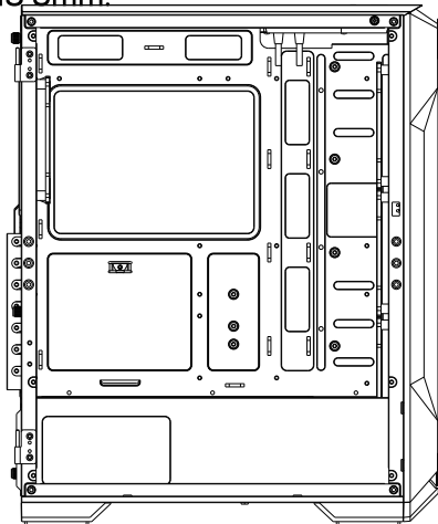
Tornillo #6-32 6.5mm
