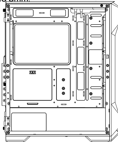
Tornillo #6-32 6.5mm
