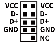
Conector USB 2.0 da Placa-Mãe
