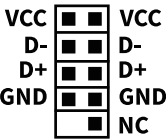
Conector USB 2.0 da Placa-Mãe
