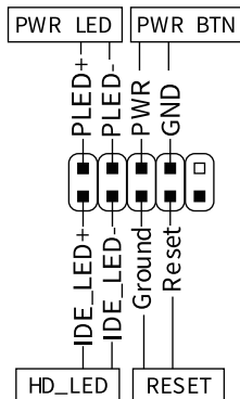
Conector Power/Reset/LED da Placa-Mãe
