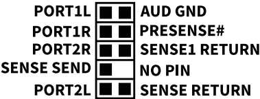
Conector de Áudio da Placa-Mãe
