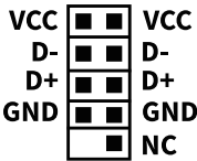
Conector USB 1.1 da Placa-Mãe
